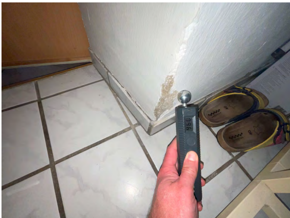
Lichtbild 14: Detail, Feuchtemessung im Bereich Teilunterkellerung an der Wandfläche, hier 96 Digits
