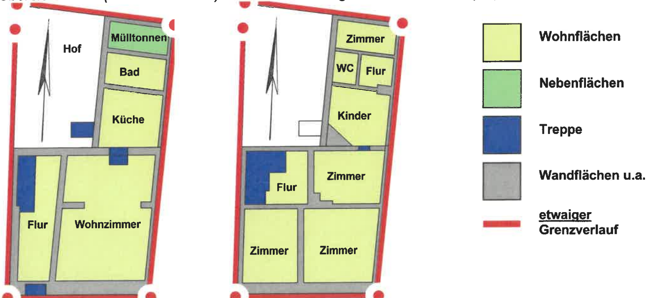
Lage- und Grundrisssskizze im Maßstab von etwa 1:200; links Erdgeschoss und rechts Obergeschoss
